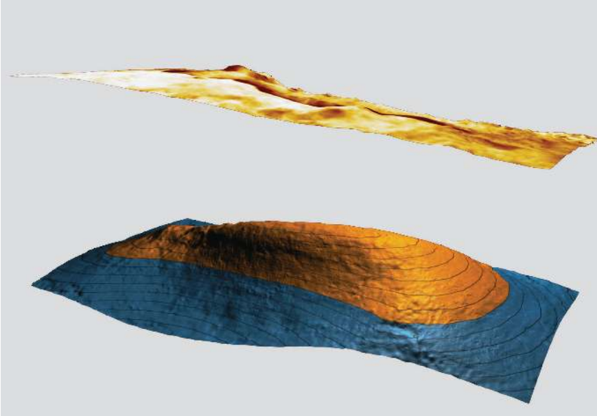
"Şahdəniz" yatağının geoloji quruluşu
